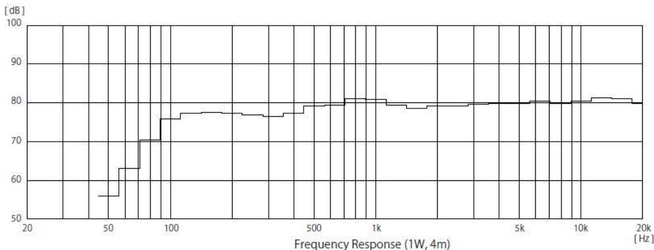
Frekvenčná charakteristika (1W/4m), 1/3 oktávové pásma
