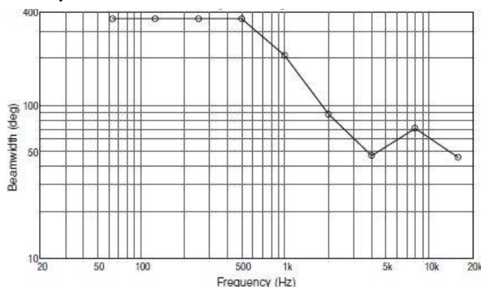
Vyžarovací uhol v závislosti od frekvencie
