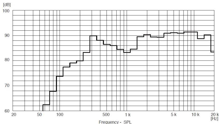
Frekvenčná charakteristika (1W/4m), 1/3 oktávové pásma
